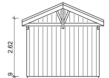
Seitenansicht rechts
