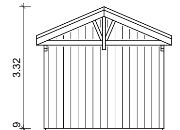
Seitenansicht links
