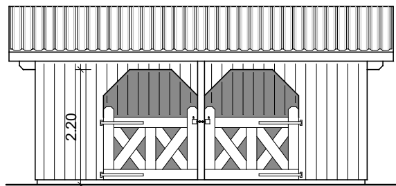
Frontansicht
