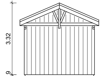
Seitenansicht links
