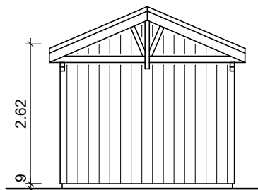
Seitenansicht rechts
