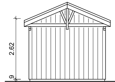
Seitenansicht rechts
