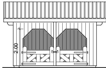
Frontansicht
